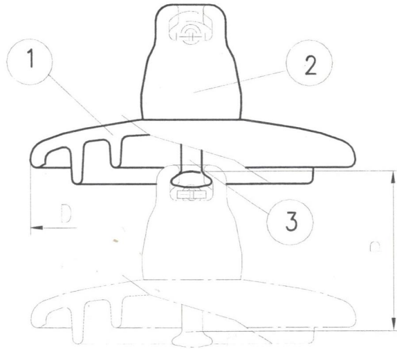
DE ACUERDO A LA ESPECIFICACION CFE 52210-02 AISLADOR DE VIDRIO TEMPLADO DESCRIPCIÓN CORTA CFE 25SVC111C
