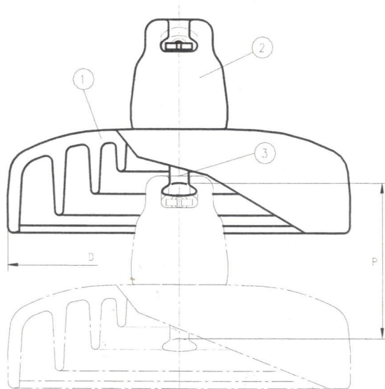
DE ACUERDO A LA ESPECIFICACION CFE 52210-02 AISLADOR DE VIDRIO TEMPLADO DESCRIPCIÓN CORTA CFE 32SVC11CM
